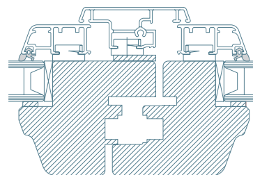
Штульп
