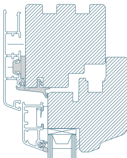
Разрез окна
