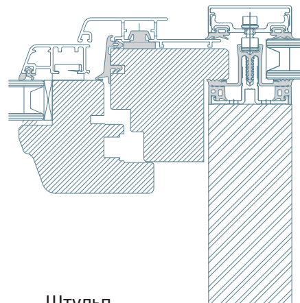
Штульп
