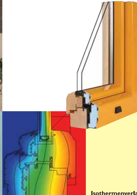
Isothermenverlauf bei MIRA-Therm
